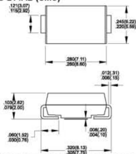
DO-214AB (SMC)
