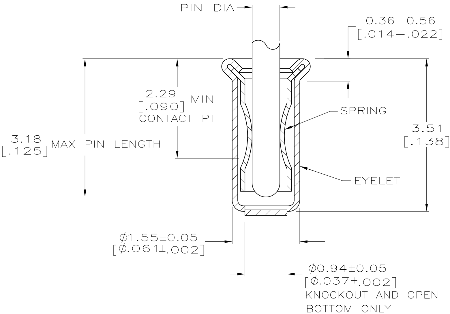
SECTION A-A
