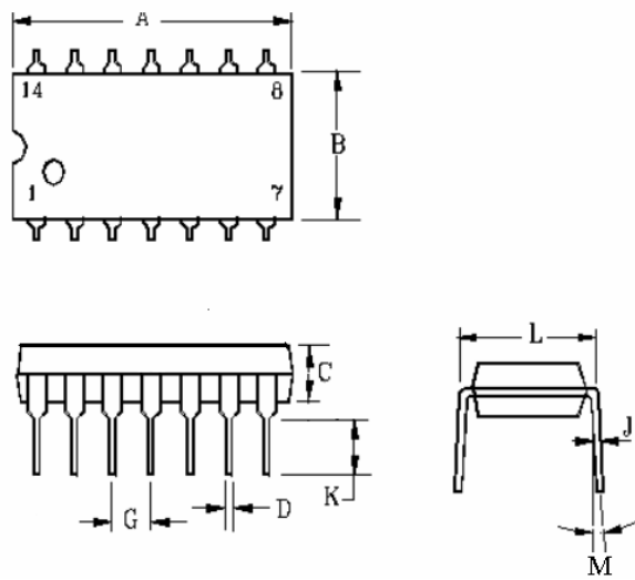
DIP-14
