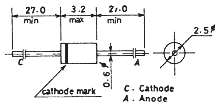
Package Dimensions 1209 (unit : mm)
