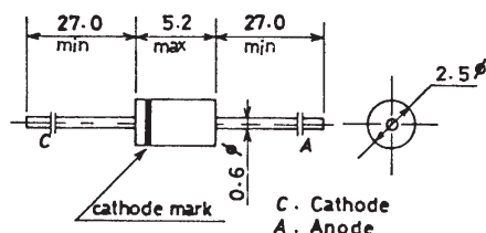
Package Dimensions 1208 (unit : mm)
