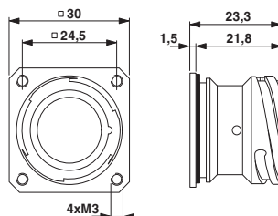
TU-00000004100 Flachdichtung
