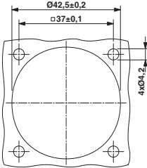
Einbaumaße
