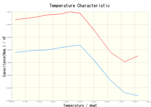
C1005X7R1C103K050BA(DC Bias = 0V)
