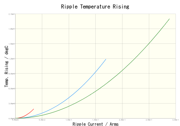
C1005X7R1C103K050BA(100kHz)
