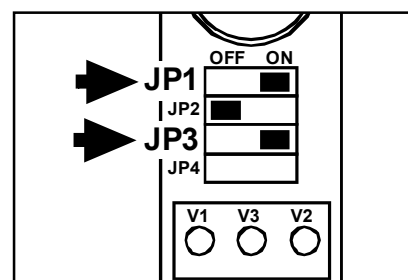
Empfänger ORRD
