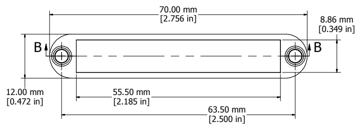
OPEN BEZEL
