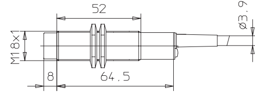
E2EL-X15M□ 2M
