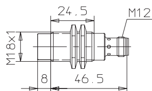
E2EL-X8M□-M1
