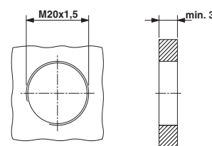
RC-00000006100, Montage Durchgangsbohrung mit Gewinde (Empfehlung bei Einbau in Stahlblechwand)
