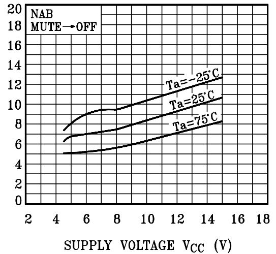
I_{CCQ} - V_{CC}
