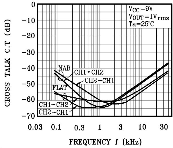
C.T - f
