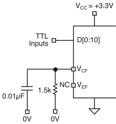
Figure 14. VCF/VEF Biasing for LVTTL Control (D) Input
