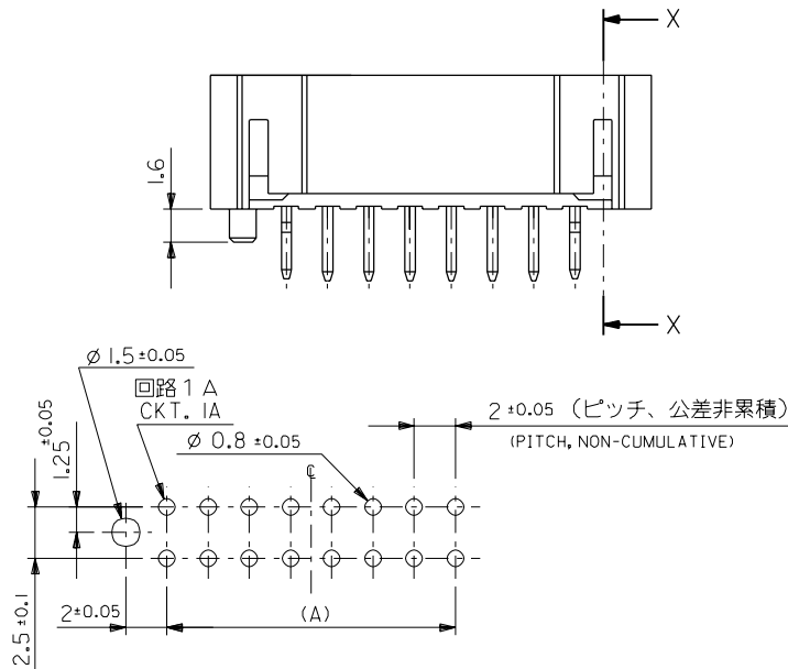
基板取付穴推奨寸法 (参考) RECOMMENDED PCB HOLE DIM.(REF.)
