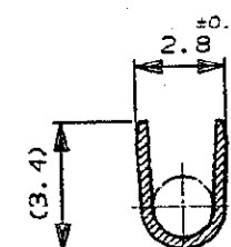
断面 A-A SECT A-A (175205のみ適用) (ONLY 175205)
