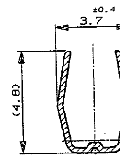
断面 B-B SECT B-B (175205のみ適用) (ONLY 175205)
