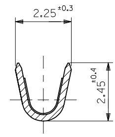
SECT.A-A
