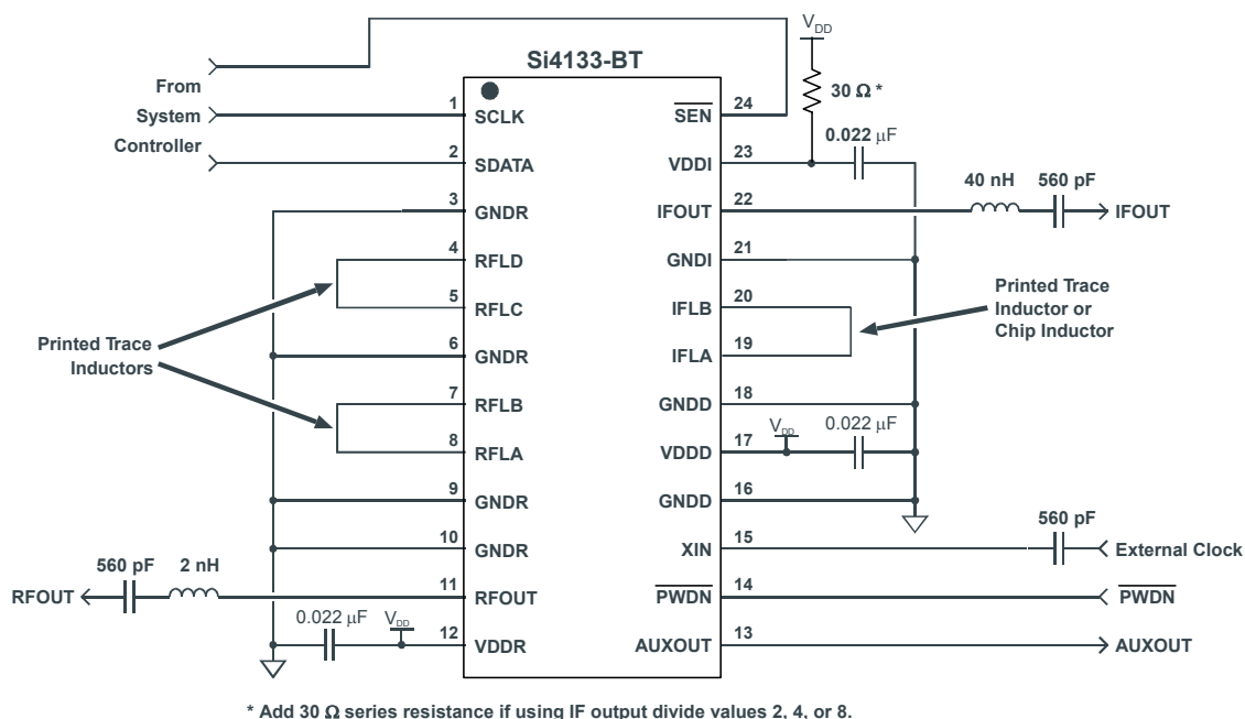
Figure 13. Si4133-BT
