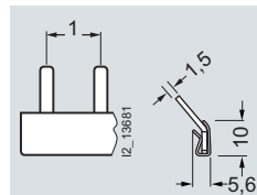
5ST3 763 5ST3 765
