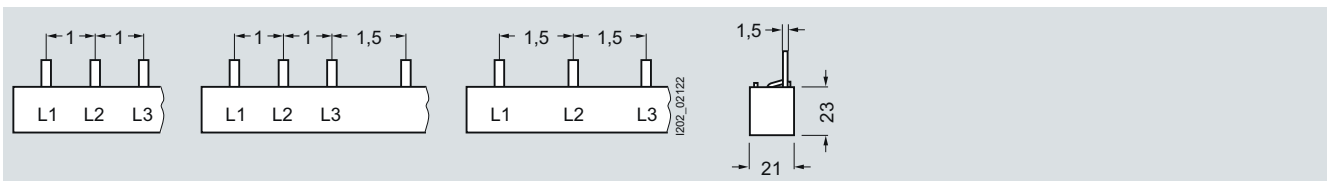
5ST3 710-0HG
