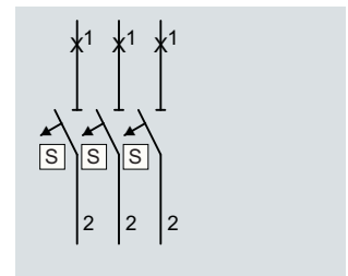
5SP3 8...-2
