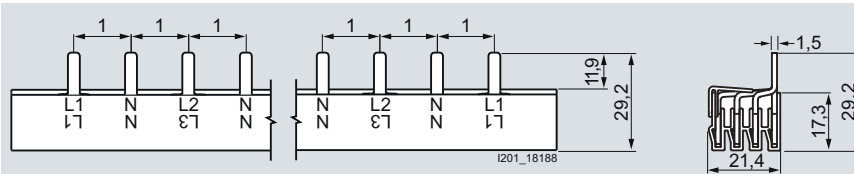
5ST3 770-3
