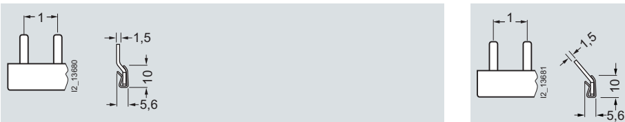
5ST3 762 5ST3 764
