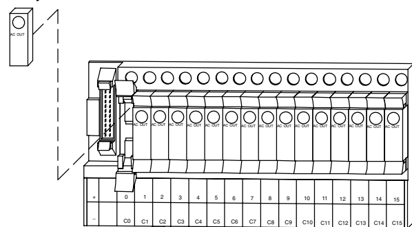
G7TC-OC16
