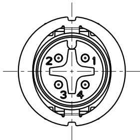
4pol A-Codierung (Steckseite) 4pole A-coding (Plug-in side)
