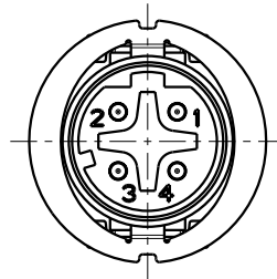
4pol D-Codierung (Steckseite) 4pole D-coding (Plug-in side)
