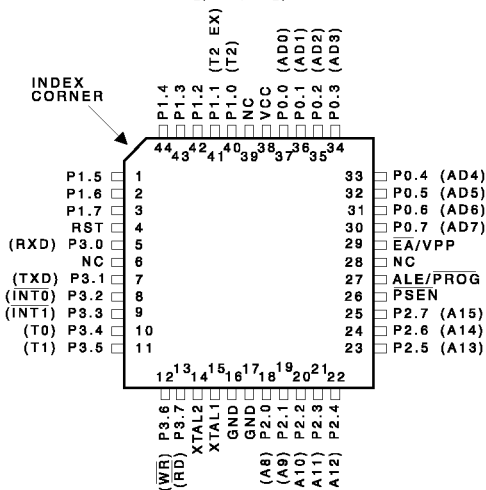
PQFP/TQFP
