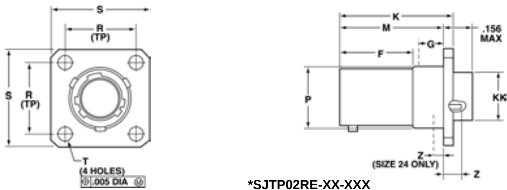
*SJTP02RE-XX-XXX
