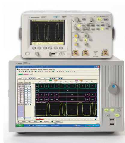
Abbildung 8. Kombinieren Sie klassenbeste Instrumente über eine einfache Verbindung
