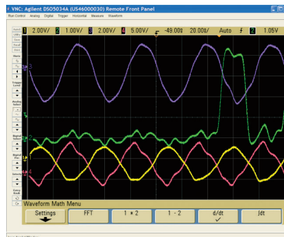
Abbildung 6. Agilent-Remote-Bedienfeld - in einem Web-Browser ausgeführt
