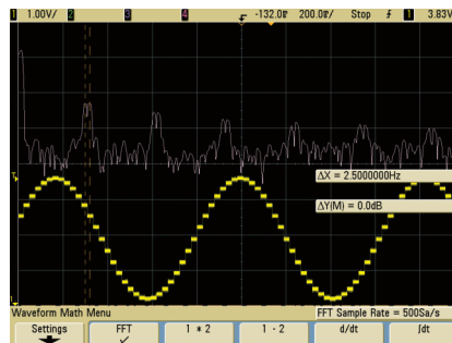
Abbildung 10. FFT ermöglicht Ihnen, den Spektralinhalt dieser ungefilterten Sinuskurve anzuzeigen
