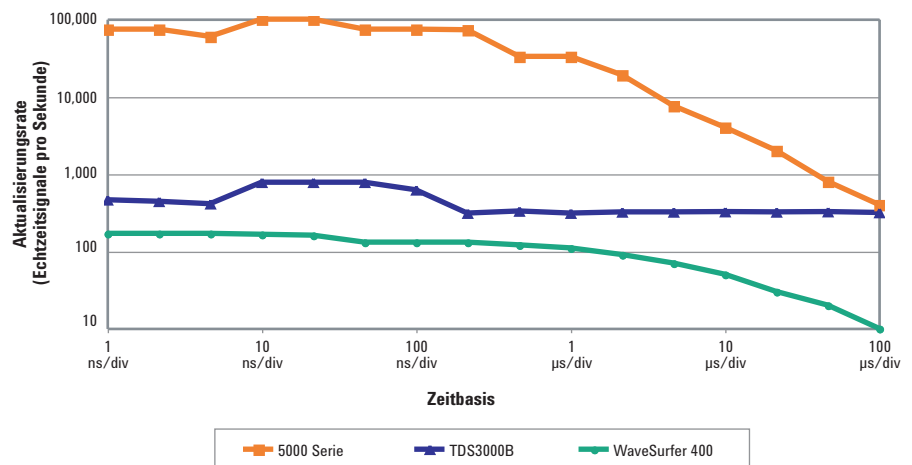
Abbildung 5. Aktualisierungsraten gängiger Oszilloskope unter Verwendung ihres standardmäßigen Zeitauffrischungsmodus in Echtzeit
