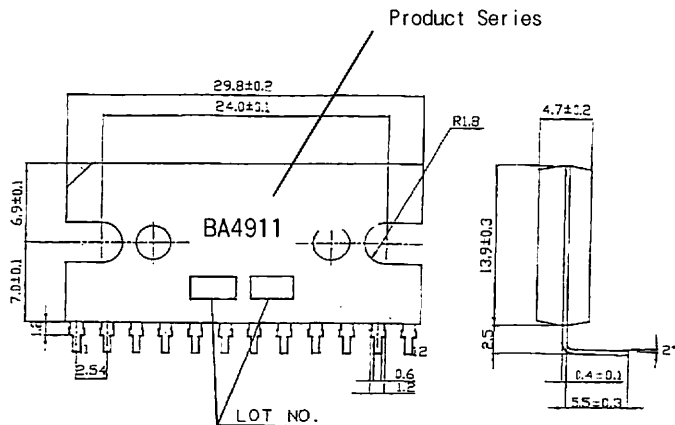
SIP-M12(V4) (Unit:mm)
