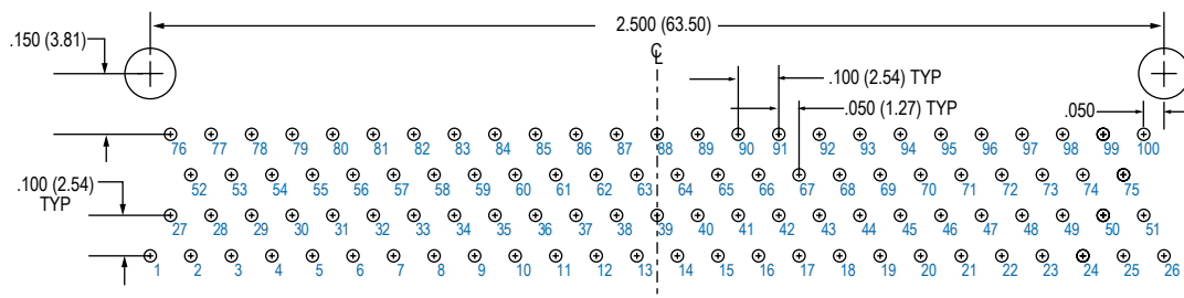
100 SOCKET
