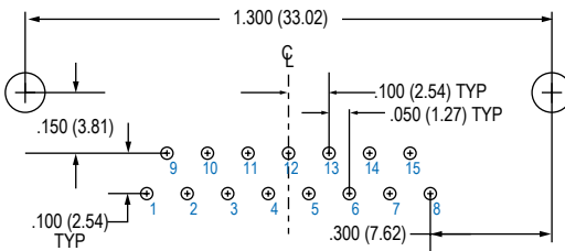
15 SOCKET
