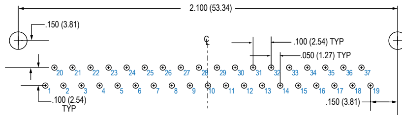
37 SOCKET
