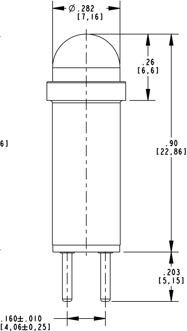
FIG. 2 (STOVEPIPE LENS)
