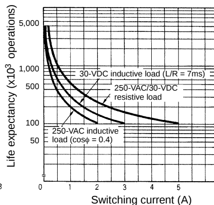
G2R-13-S, G2R-1A3-S
