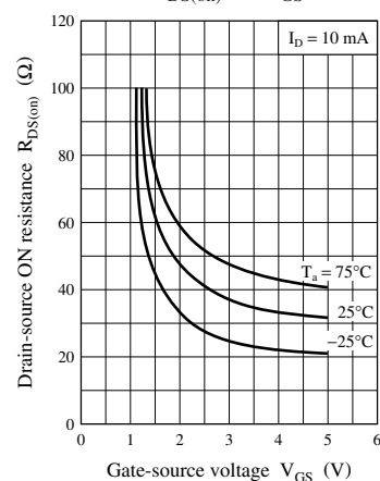
R_{DS(on)} - V_{GS}
