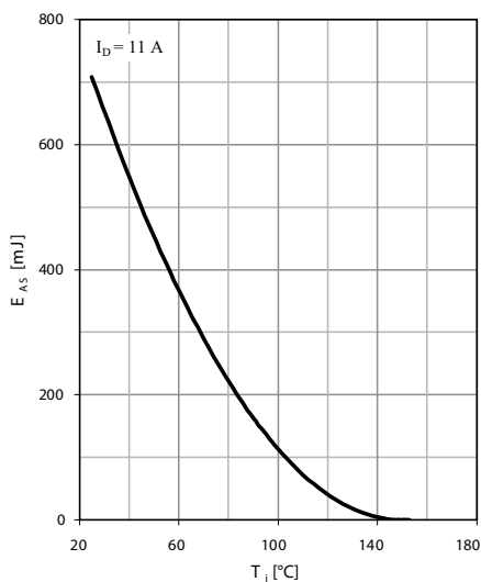
Fig. 10 Avalanche energy
