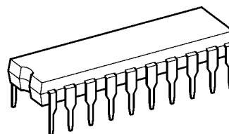
DIP20-P-300-2.54A
