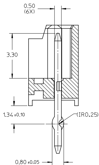
SECTION D-D
