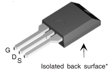
ISOPLUS 220LV™
