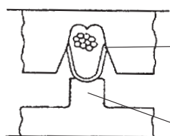
Die geschrägten Außenflanken dienen der besseren Führung der Crimphülse in der Obermatrize als auch dem besseren Einrollen der Crimphülsenflanken
