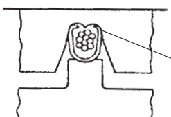
Obermatrize und die sich einrollenden Crimphülsenflanken zwingen das abisolierte Leiterende in den Crimphülsenboden
