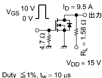
図 6.2.1 スwitchング時間の測定回路例
