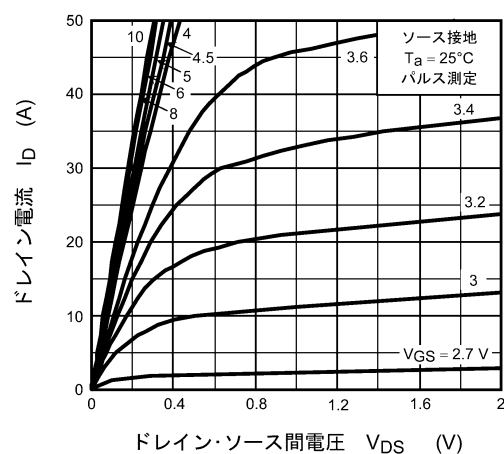
図 8.2 I_D - V_{DS}
