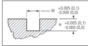
Groove Dimensions
