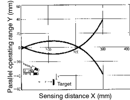
E32-T11L with E39-F3 and E3X-NH amplifier
