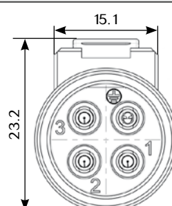
Wiring face
