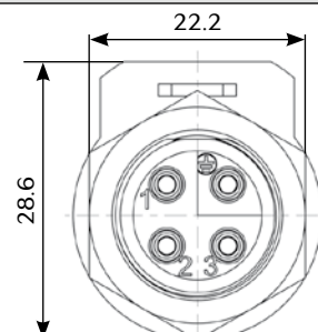
Wiring face
