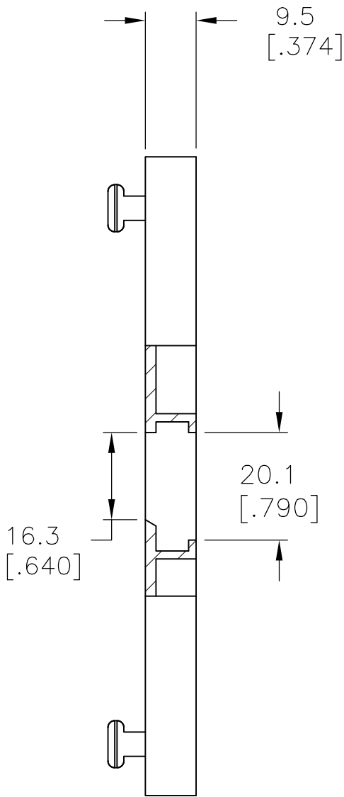
SECTION A-A
