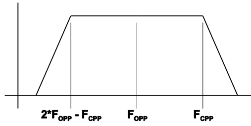
Polyphase Band-pass Filter for OOK
