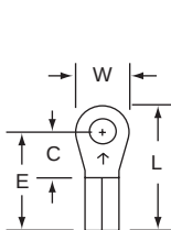
12-4S Stud Size 4 Wire Range 16-14
