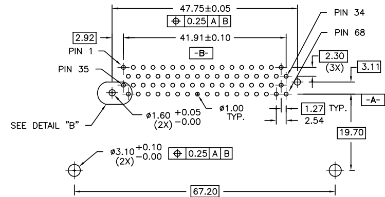
P.C.B. LAYOUT
