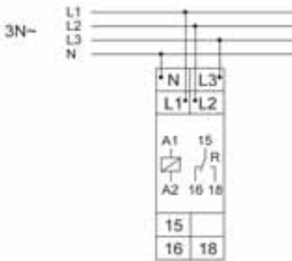
Wiring E236-US 1.1D
