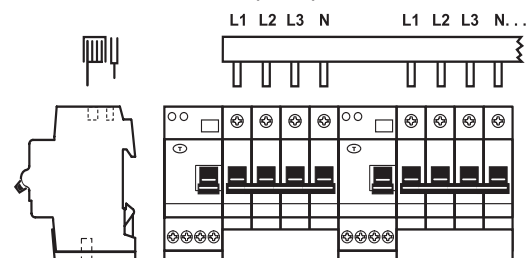
PS 4/40/16-DDA 204 T DS 204 ( \leq 40 A) + DS 204 ( \leq 40 A) + DDA 204 ( \leq 40 A) + S 204 + DDA 204 ( \leq 40 A) + S 204 ...
