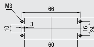
Montageausschnitt Panel cut-out
