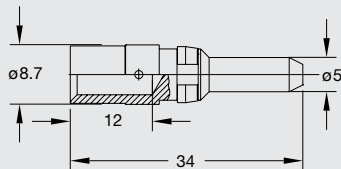
Stiftkontakt/Pin contact
