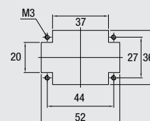
Montageausschnitt Panel cut-out
