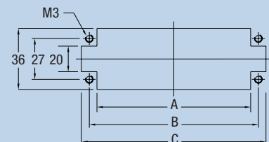
Montageausschnitt für Kontakteinsätze bei Verwendung ohne Gehäuse
