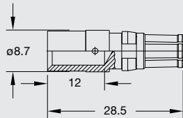
Buchsenkontakt/Socket contact
