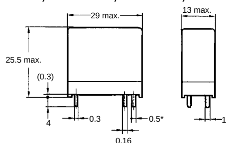
G2R-1A
