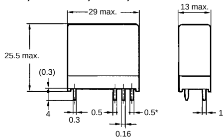
G2R-1
