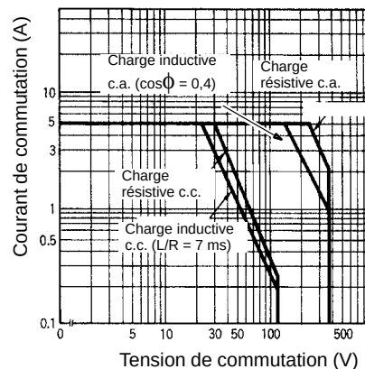
G2R-1Z, G2R-1AZ
