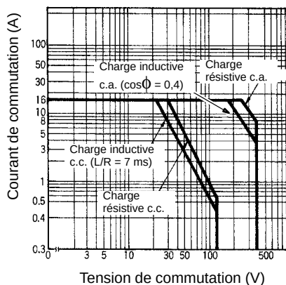
G2R-1-E, G2R-1A-E
