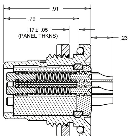
SECTION A-A SCALE 3.000
