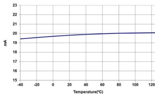
lin (Dyn)
