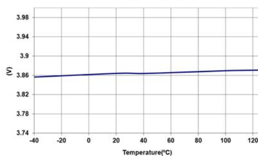
Vcc_UVLO_Stop
