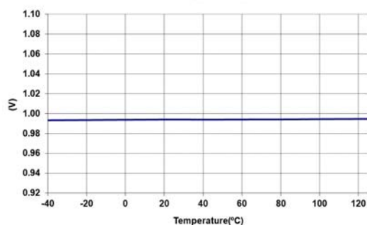
Enable_UVLO_Stop
