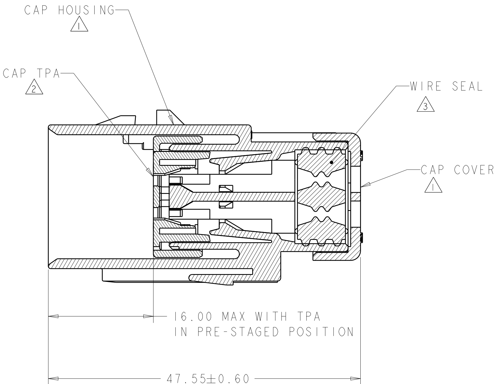
SECTION A-A
