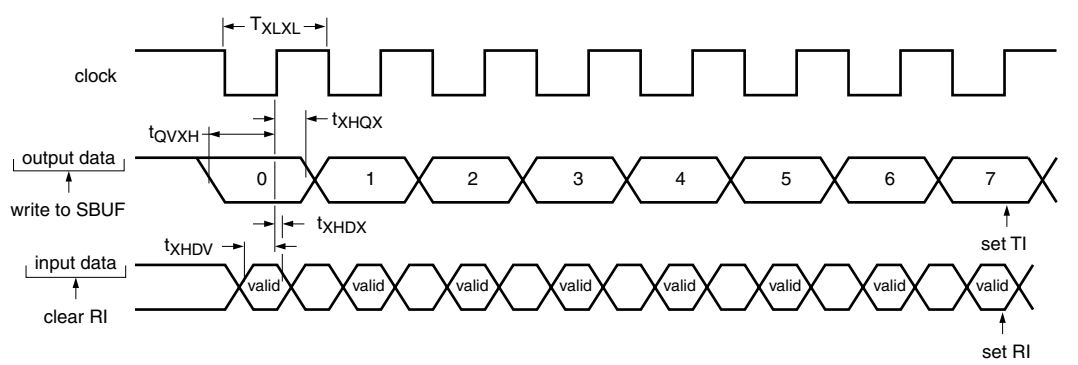
Fig 23. Shift register mode timing
