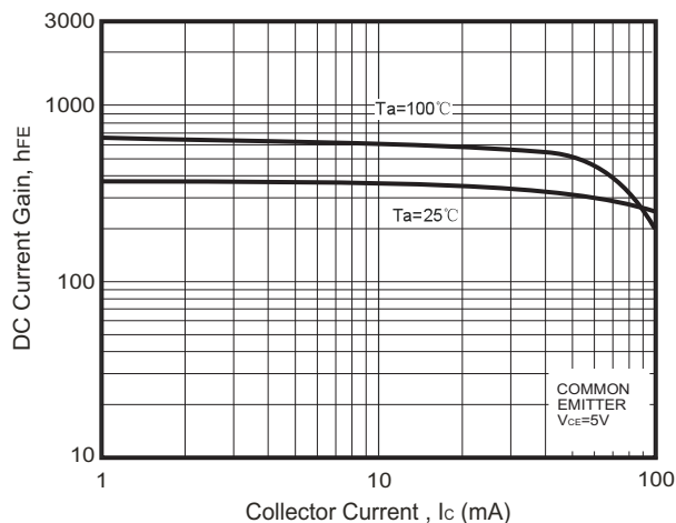
Fig.2 - h_{FE} - I_C
