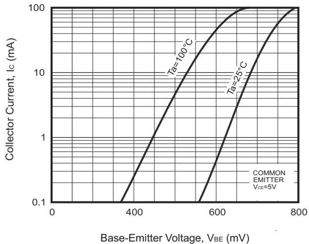
Fig.5 - I_C - V_{BE}
