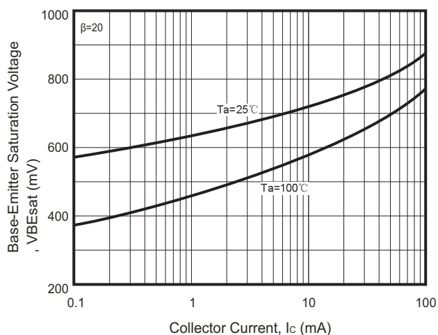
Fig.3 - V_{BEsat} - I_C
