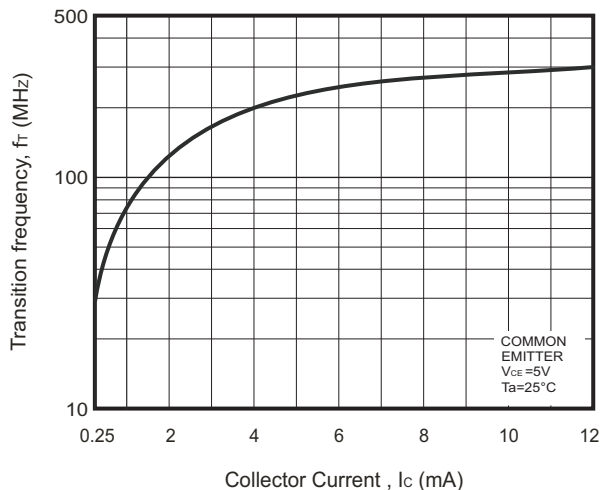
Fig.6 - f_T - I_C
