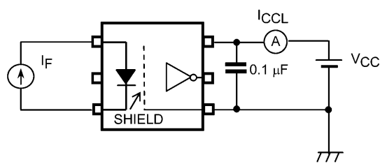
図 12.1.4 I_{CCL} 測定回路
