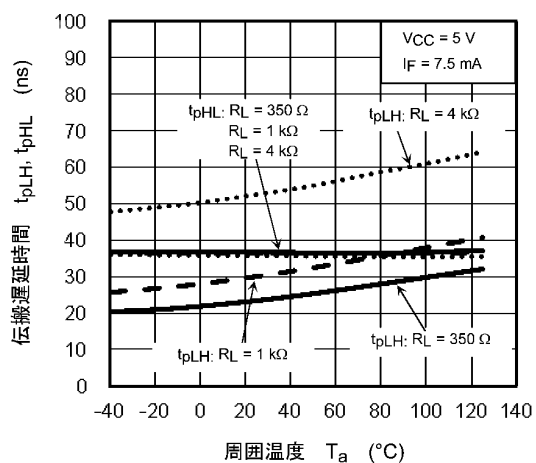
図 12.2.11 t_{pLH} / t_{pHL} - T_a
