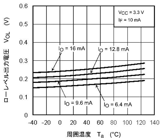
図 12.2.4 V_{OL} - T_a
