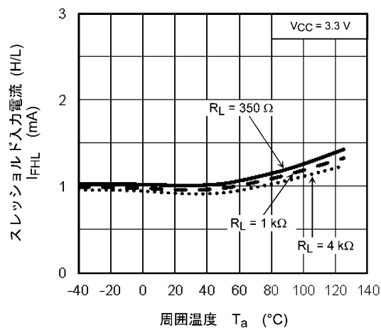
図 12.2.8 I_{FHL} - T_a
