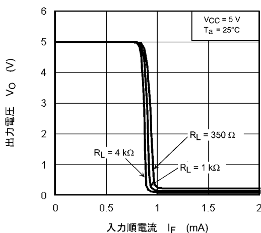
図 12.2.5 V_O - I_F
