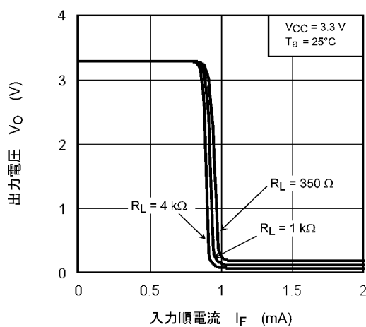
図 12.2.6 V_O - I_F
