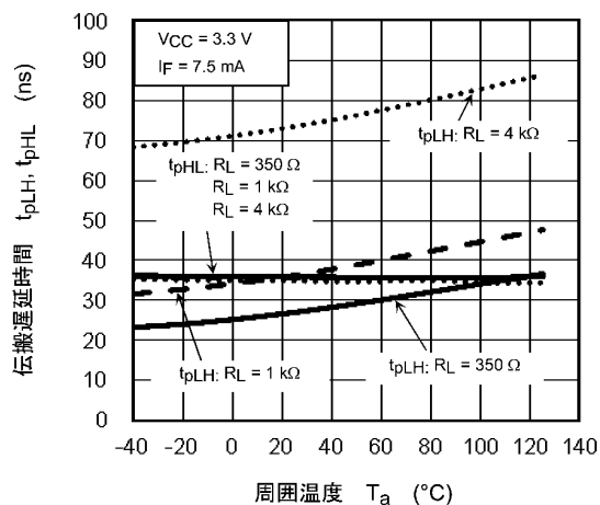
図 12.2.13 t_{pLH} / t_{pHL} - T_a
