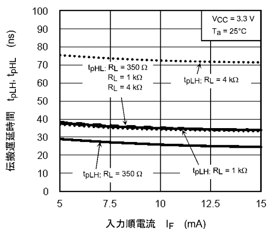
図 12.2.17 t_{pLH} / t_{pHL} - I_F
