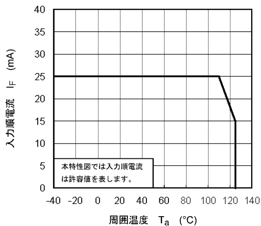
図 12.2.2 I_F - T_a
