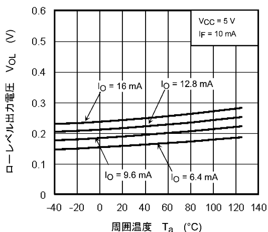
図 12.2.3 V_{OL} - T_a
