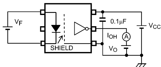
図 12.1.1 I_{OH} 測定回路
