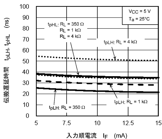
図 12.2.15 t_{pLH} / t_{pHL} - I_F
