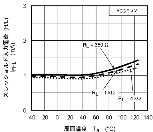
図 12.2.7 I_{FHL} - T_a
