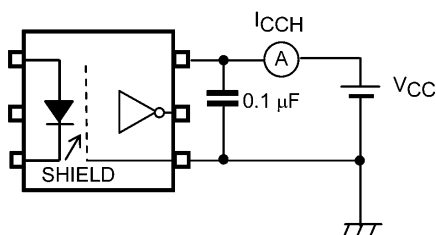
図 12.1.3 I_{CCH} 測定回路
